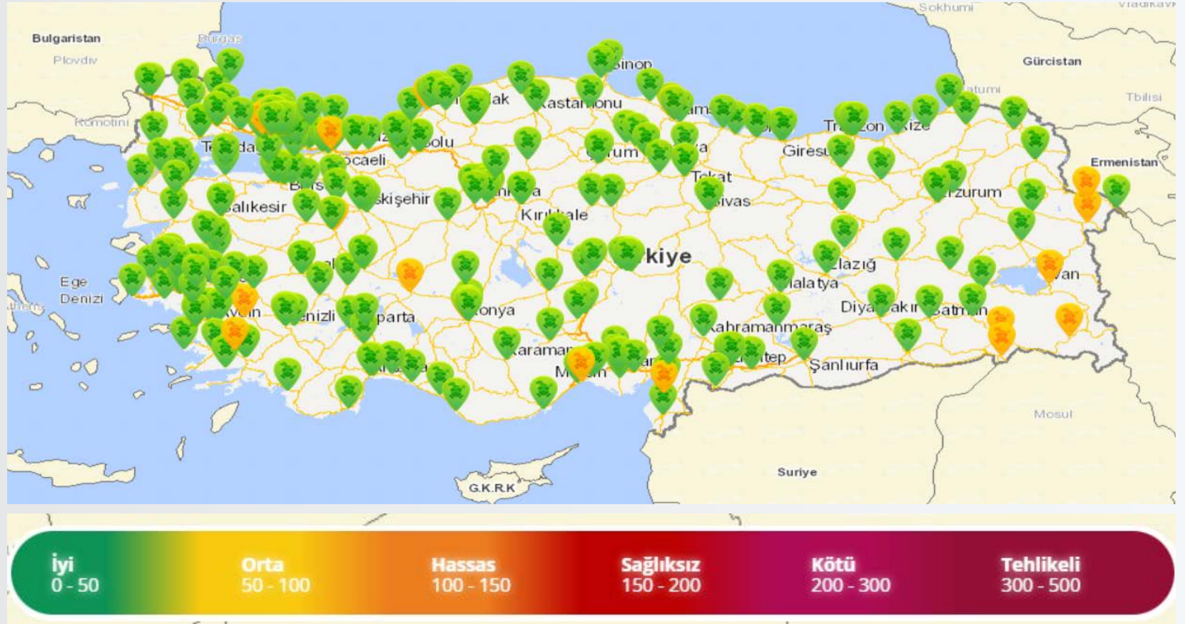
Türkiye Hava Kirliliği Haritası T.C. Çevre , Şehircilik ve İklim Değişikliği Bakanlığı 20.03.2025 verileri
